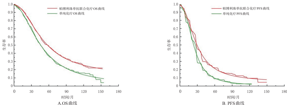
图4 ITT亚组两种治疗方案拟合前后的KM曲线
