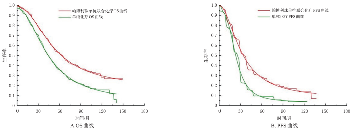
图3 PD-L1 CPS ≥ 10分亚组两种治疗方案拟合前后的KM曲线
