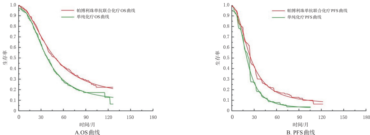
图2 ESCC亚组两种治疗方案拟合前后的KM曲线
