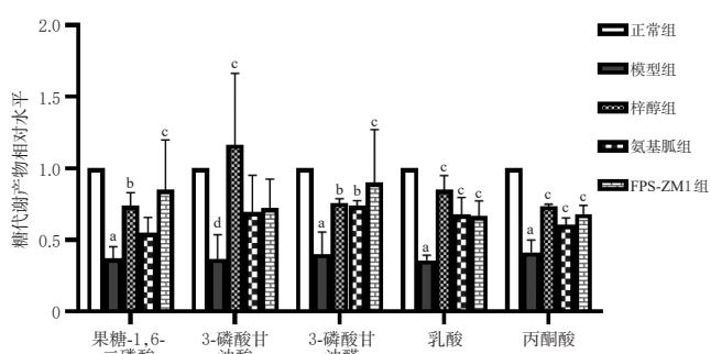
图 3 梓醇对 KK-Ay 自发性糖尿病小鼠睾丸组织中糖代谢产物水平的影响( \bar{x} \pm s, n=6 )
