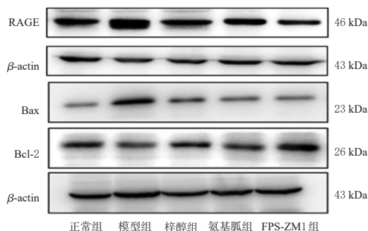
图 5 各组小鼠睾丸组织中 RAGE、Bax 和 Bcl-2 蛋白表达的电泳图
