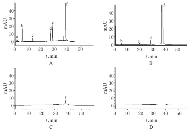
图1 系统适用性试验高效液相色谱图
